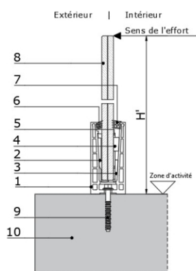
Figure 3 – GlassFit SV-1403 Top – Montage au sol et Montage au sol surélevé
