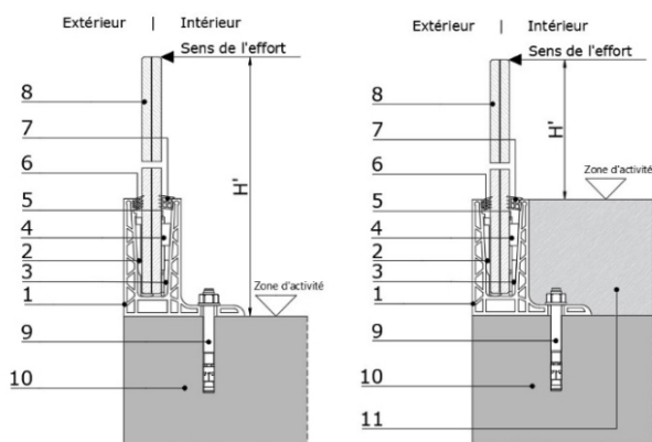
Figure 3 – GlassFit SV-1403 Top – Montage au sol et Montage au sol surélevé
