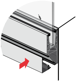
SV-1704 Side Cladding CL-1704-1
