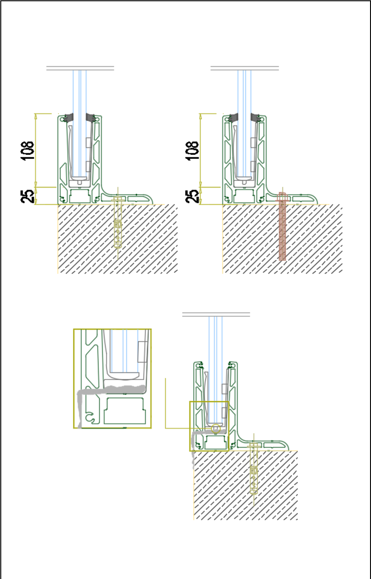
Détail Profil KF1050 (Fixation non testée)
