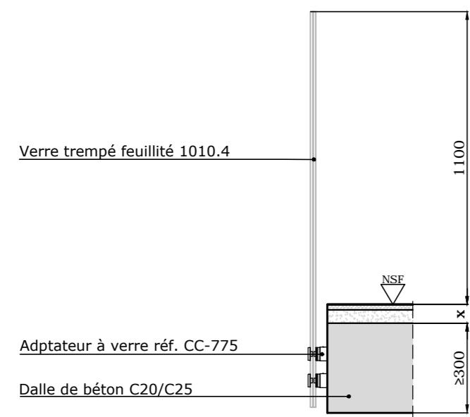
Coupe A-A GlassFit CC-775 Sans main-courante Échelle 1:20
