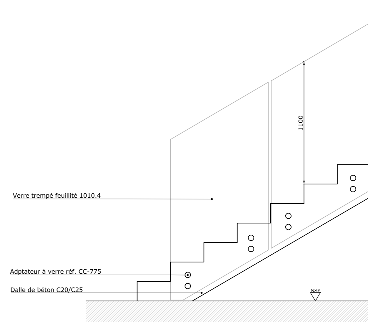
Détail de début d'escalier GlassFit CC-775 Sans main-courante Échelle 1:20
