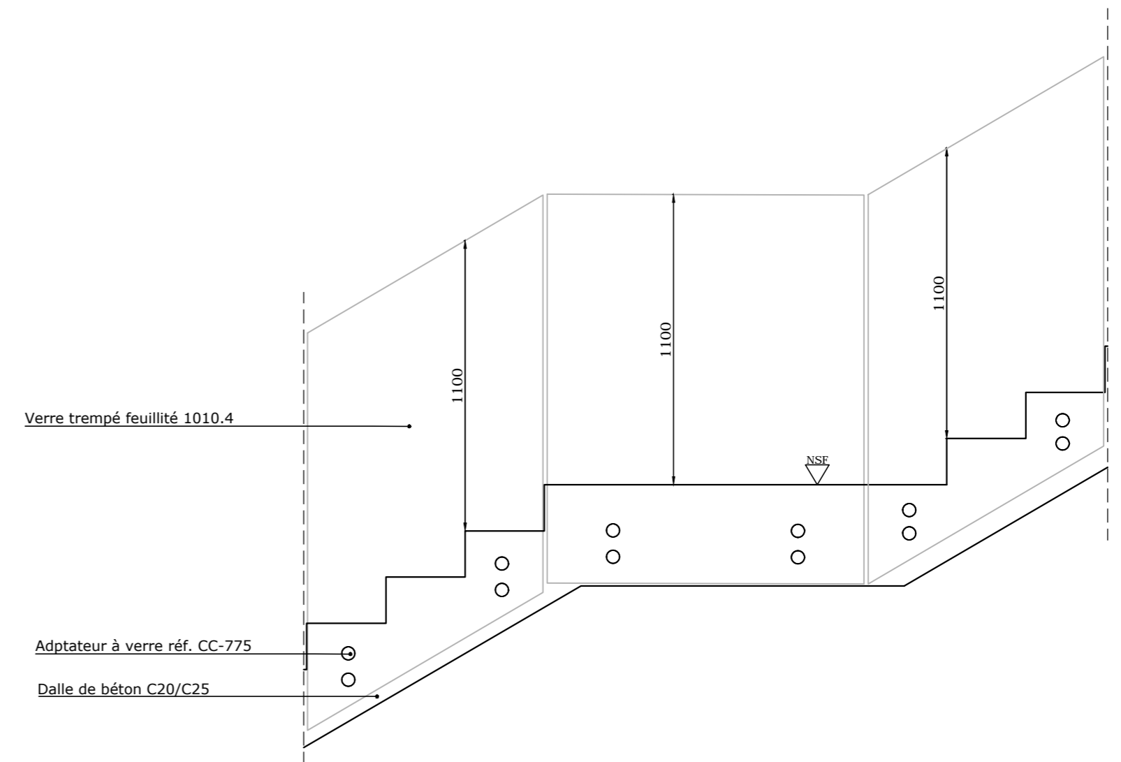
Détail jonction tronçons inclinés avec tronçons horizontals GlassFit CC-775 Sans main-courante Échelle 1:20
