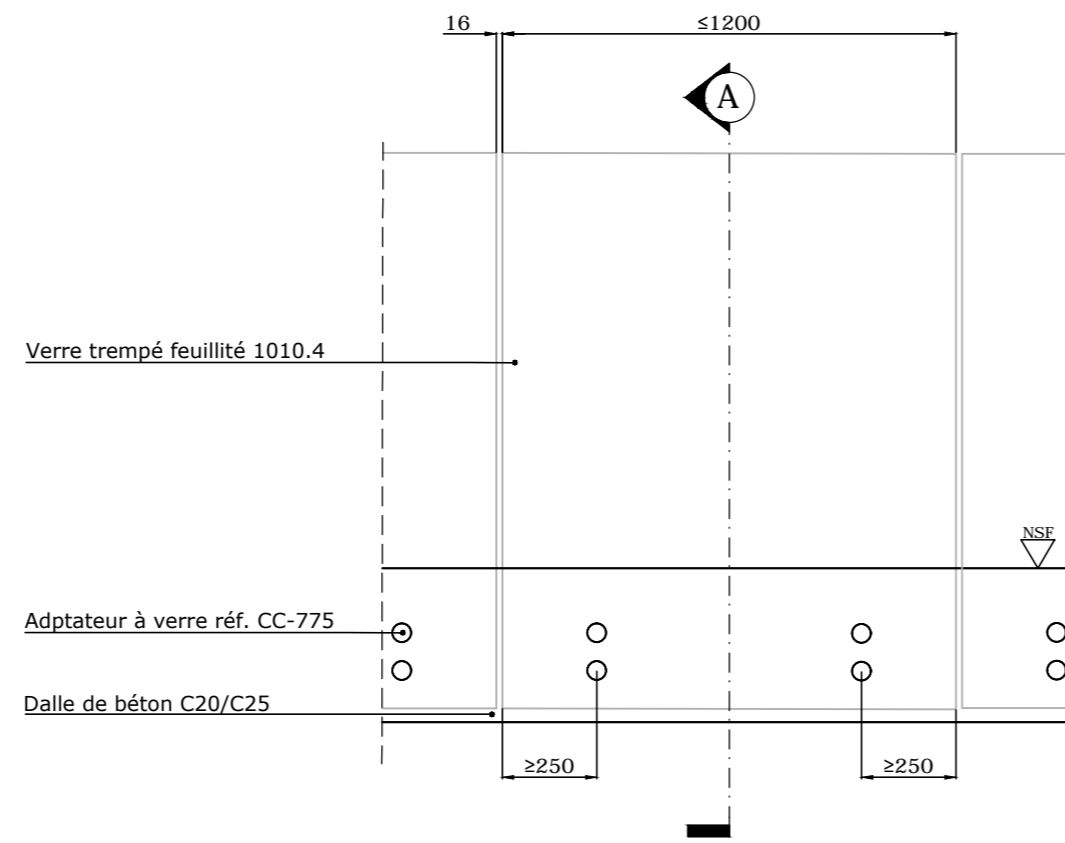
Détail tronçon horizontal type GlassFit CC-775 Sans main-courante Échelle 1:20
