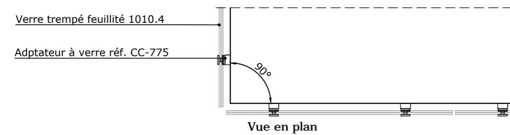
Détail de jonction à l'angle GlassFit CC-775 Sans main-courante Échelle 1:20
